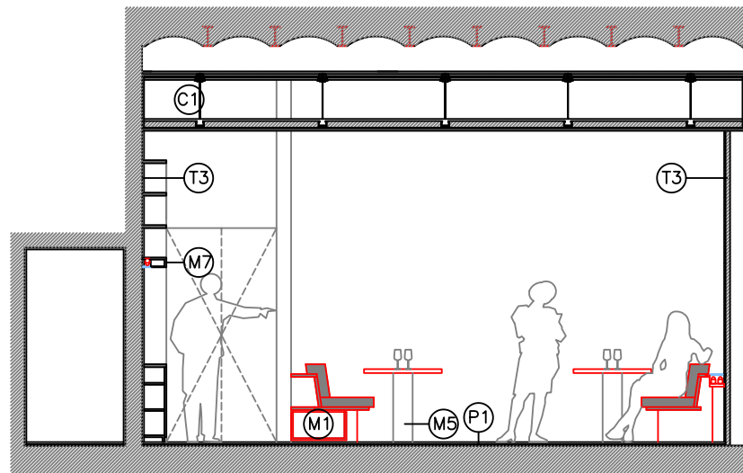
SECCIÓ 6-6
