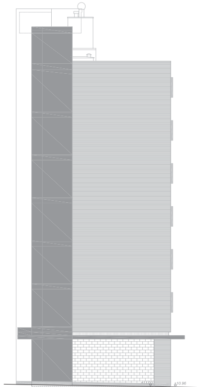
BLOQUE TIPO (BLOQUE 2), ALZADO LATERAL 2
