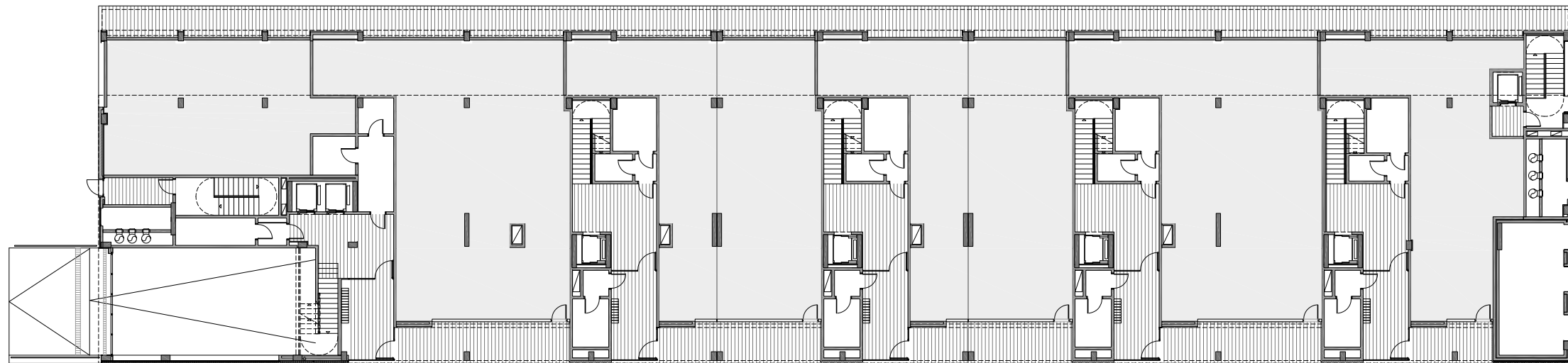
⊖ PLANTA BAJA 1:300
