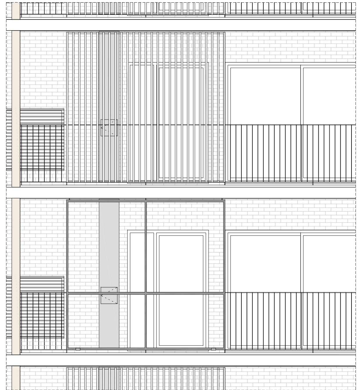
ALÇAT
