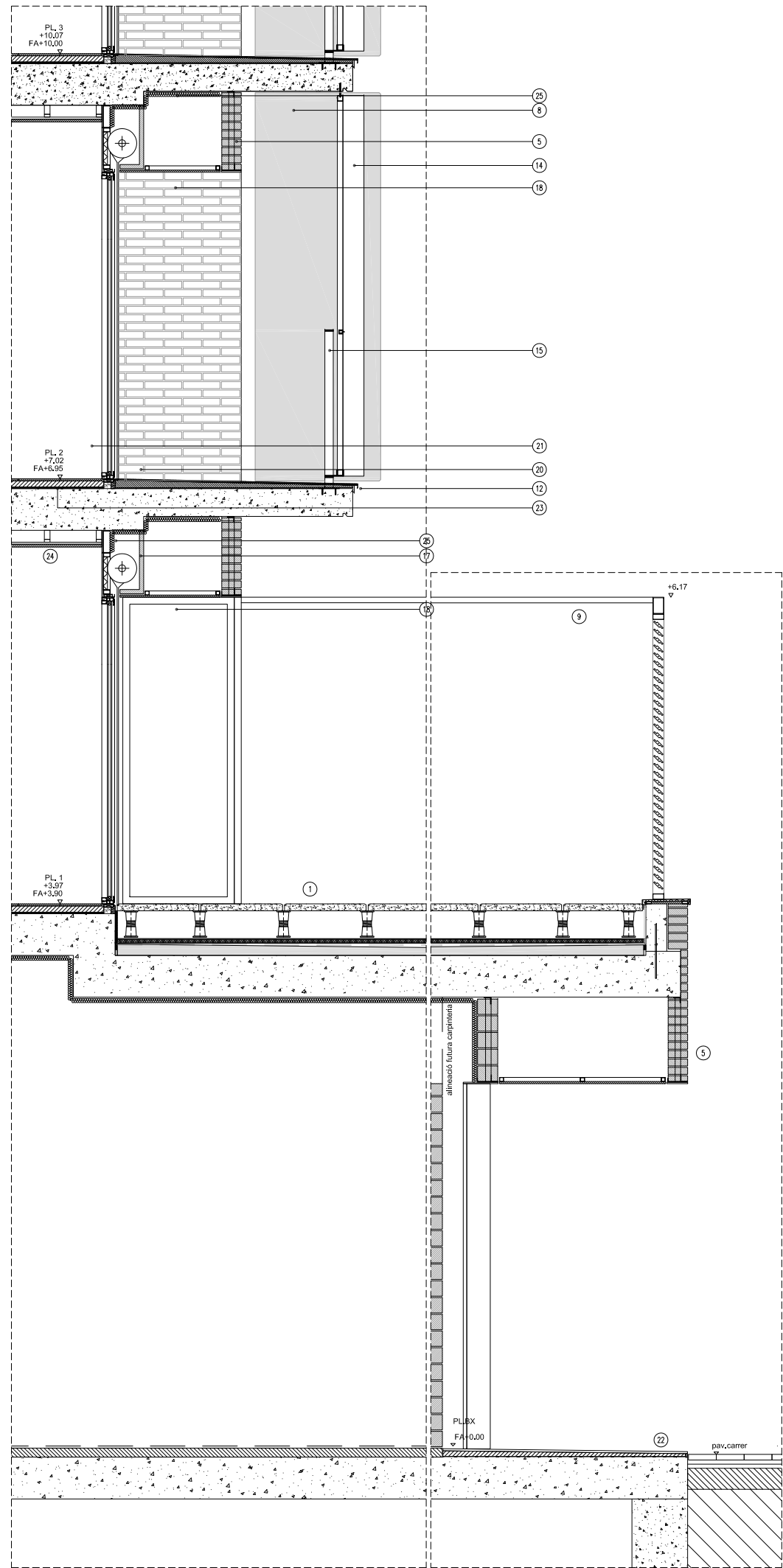
SECCIÓ CONSTRUCTIVA
