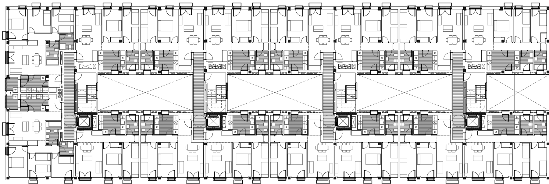
PLANTA TIPO (2ª A 4ª)
