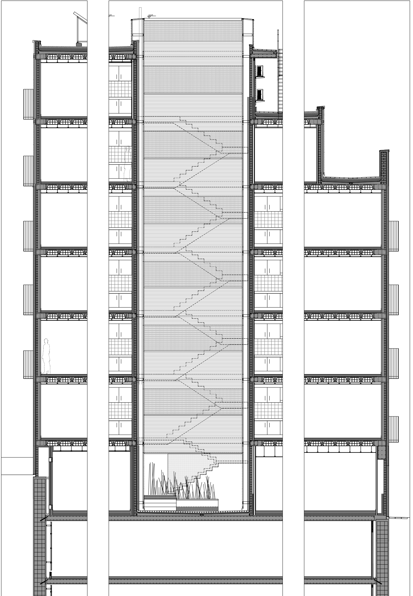
SECCION TRANSVERSAL POR MUROS
